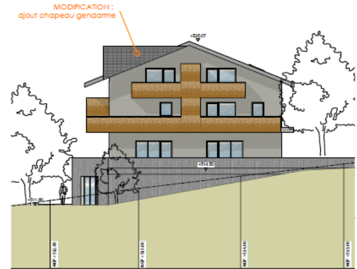
BATIMENT D - FACADE EST
