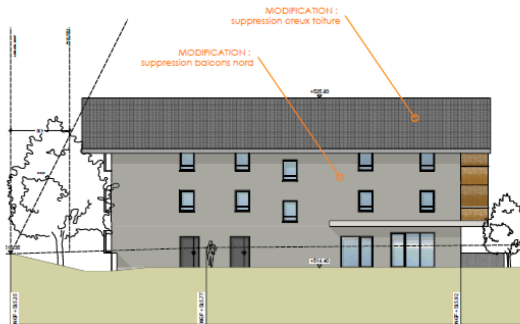
BATIMENT E - FACADE NORD
